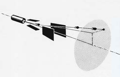
Fig. 8. Elektrische afbuiging in twee richtingen
