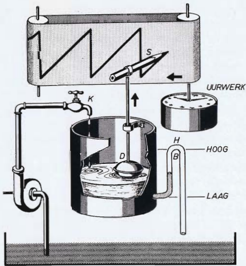
Fig. 15. Een hydraulische zaagtandgenerator
