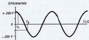
Fig. 13. Grafiek van een wisselspanning
