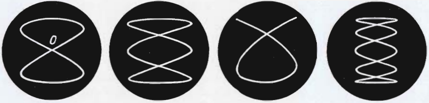
Fig. 12. Figuren van Lissajous
