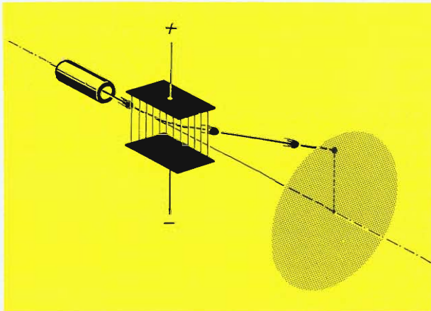
Fig. 7. Verticale afbuiging van een elektronenstraal door een elektrisch veld
