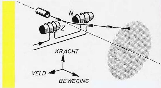
Fig. 9. Magnetische afbuiging
