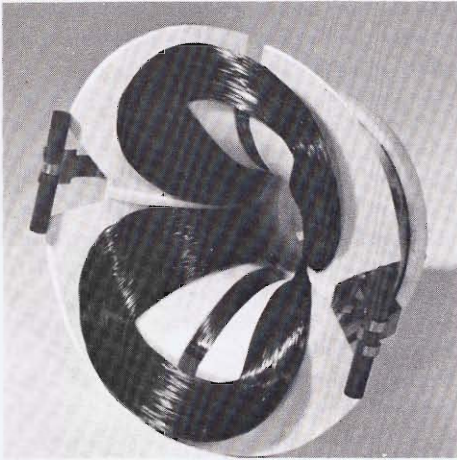
Fig. 10. Spoelensysteem van een beeldbuis
